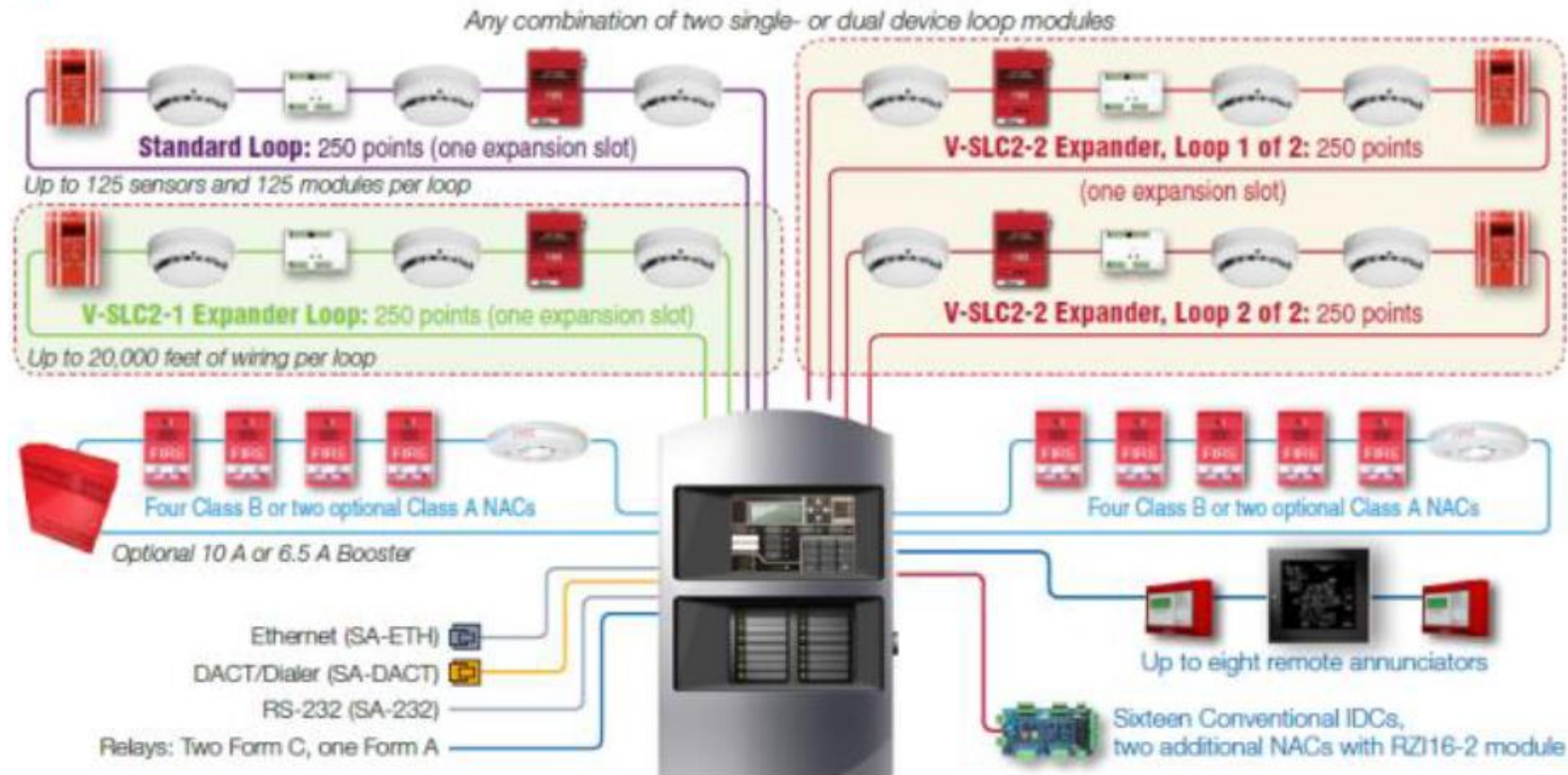
ESQUEMA EJEMPLO DE INSTALACION DE SISTEMA DE DETCCION DE INCENDIOS EDWARDS
